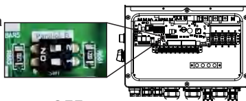
Figura 3.22 Conexão do terminal paralelo
