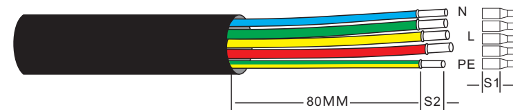
Figura 5.17 Decapagem do cabo CA
